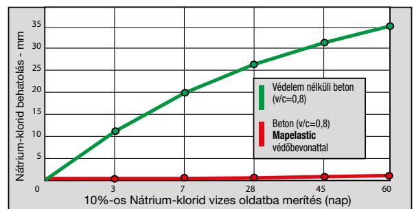
3. ábra: Mapelastic védőbevonat porózus betonon nátrium-klorid behatolás ellen
