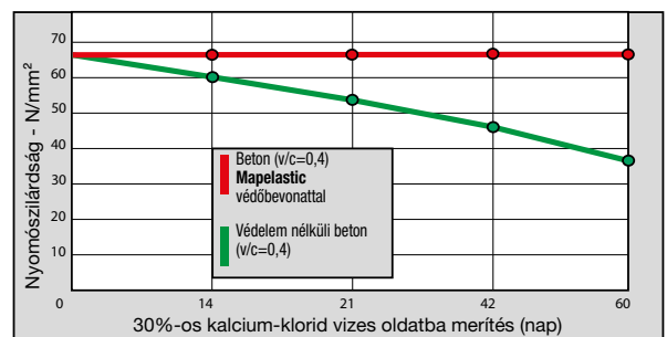
4. ábra: Mapelastic védőbevonat a kalcium-klorid alapú útszóró sók okozta mechanikai szilárdság csökkenés ellen
