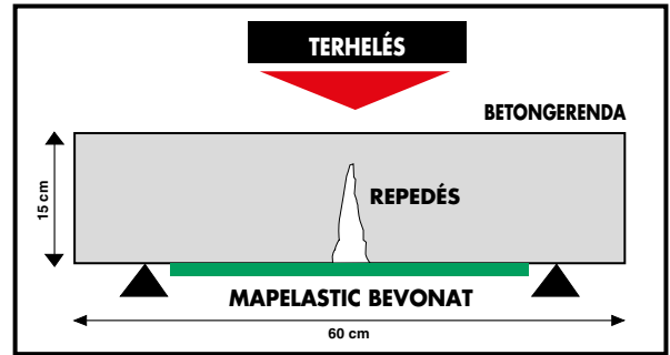
1. ábra: Hajlító igénybevételnek kitett betongerenda alsó oldali hajszálrepedésének védelme Mapelastic-kal
