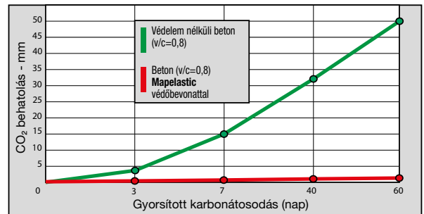
2. ábra: Porózus beton gyorsított (30% CO 2 ) karbonátosodás elleni védelme Mapelastic-kal
